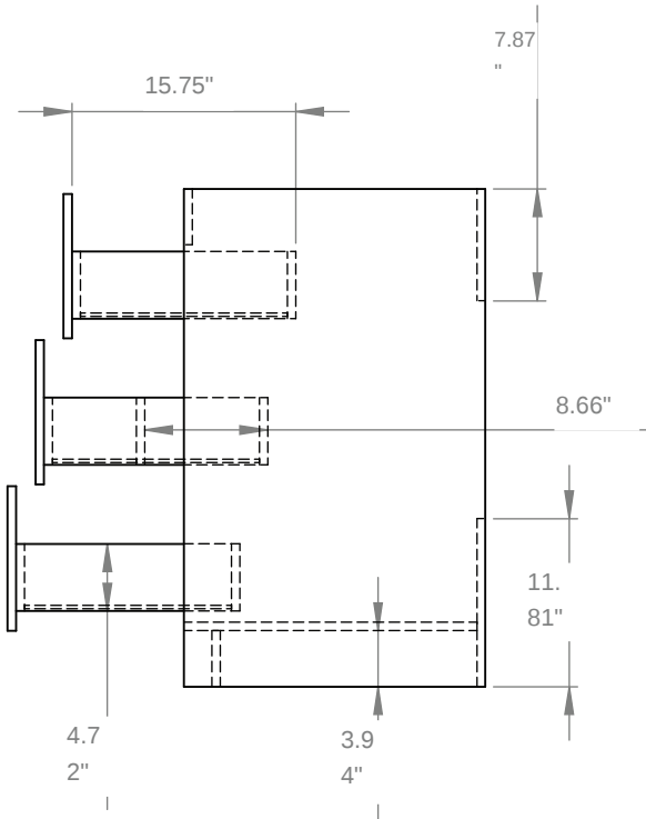
VUE LATÉRALE
