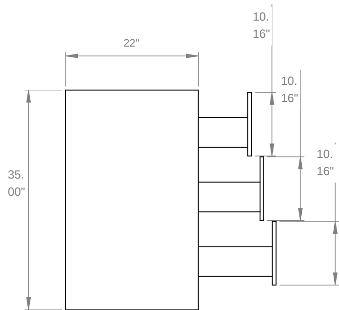
VUE LATÉRALE
