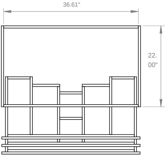
VISTA SUPERIOR
