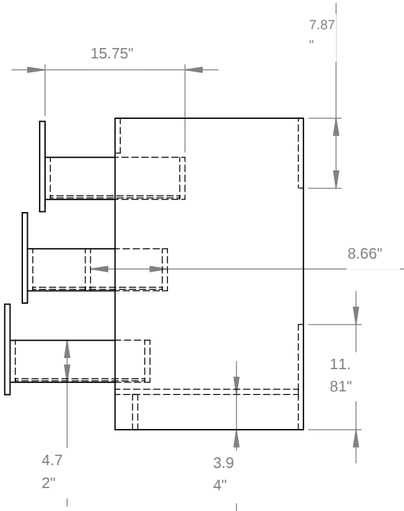
VISTA LATERAL
